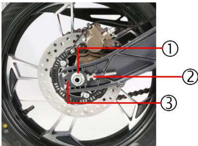
Holgura o juego libre de la cadena: 18-25 mm
