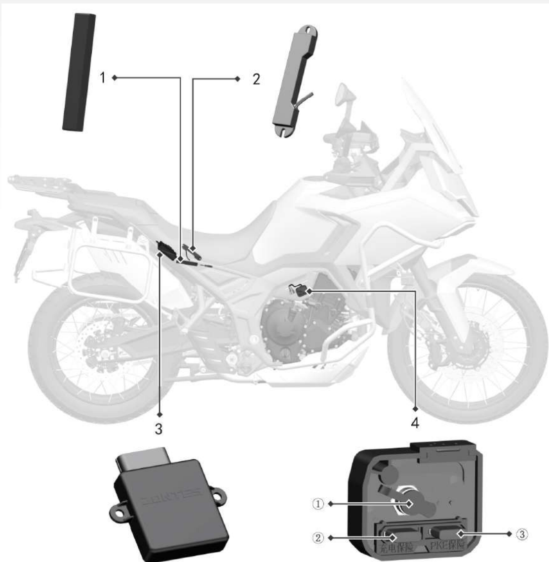
Zona sensible de la antena 3D
