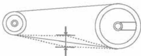
Holgura o juego libre de la cadena: 18-25 mm
